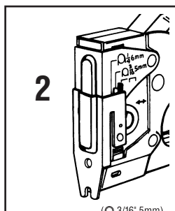
Fig. 2: Position intermédiaire pour fixer des fils et câbles plus fins.
